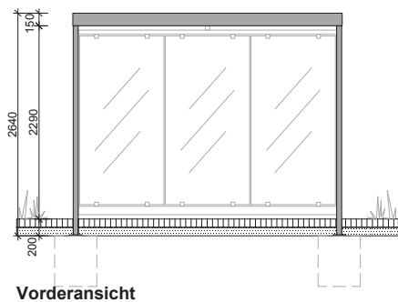
Vorderansicht
