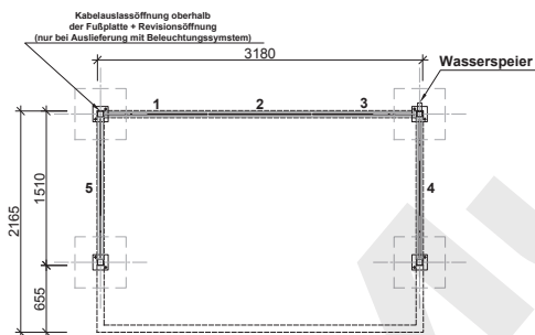
Grundriss
